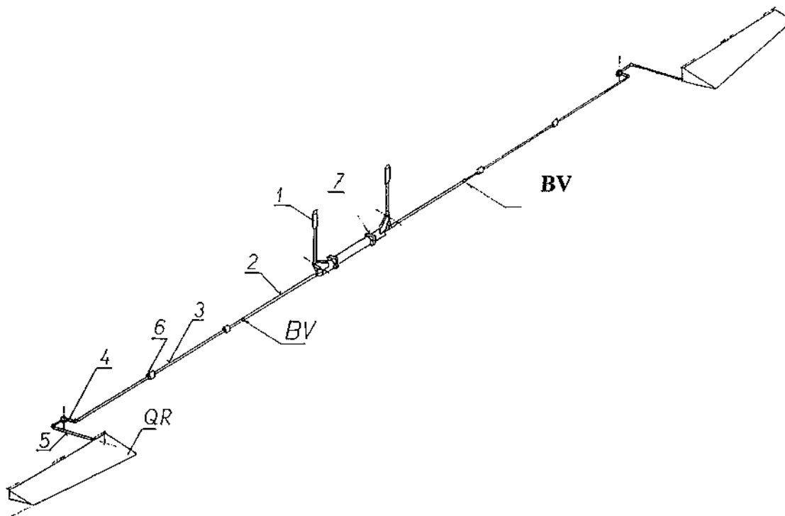
Fig....Système de contrôle latéral
