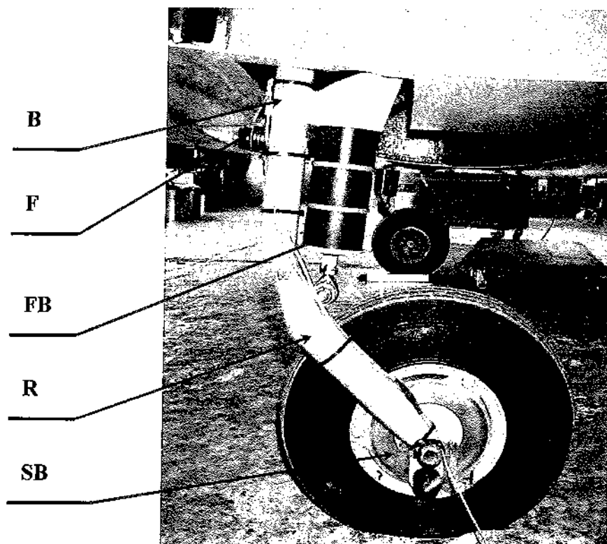
Fig.... Jambe principale du train rétractable
